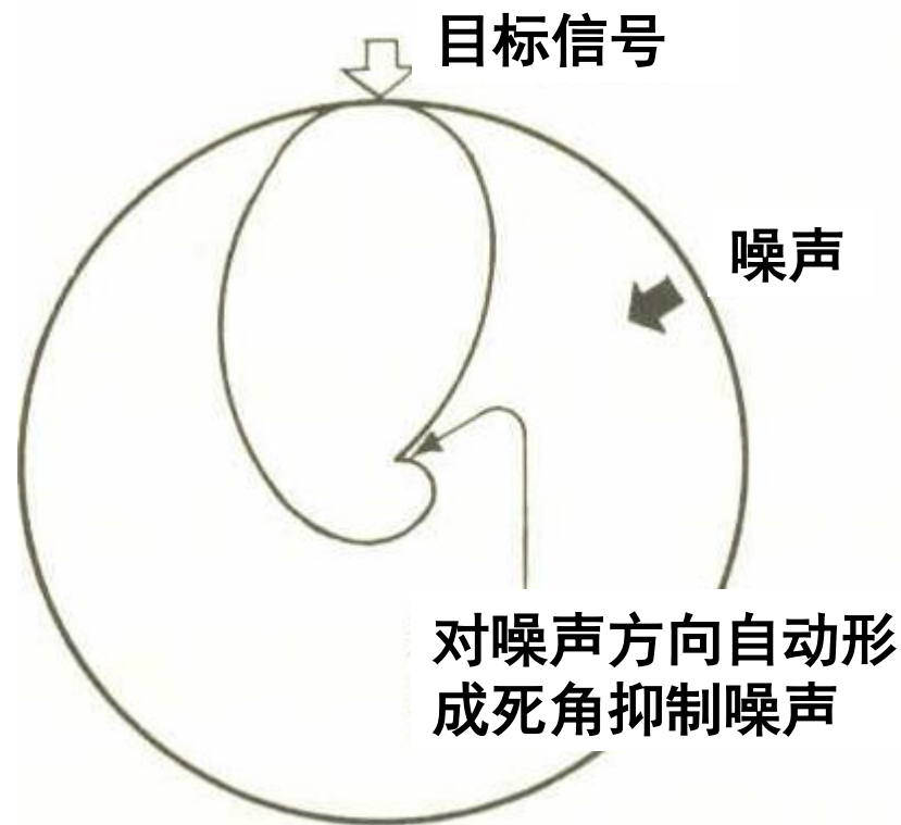
自适应波束形成
