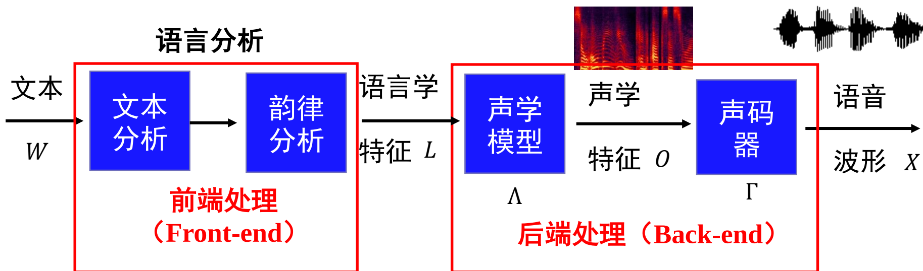
统计参数语音合成的框架图
