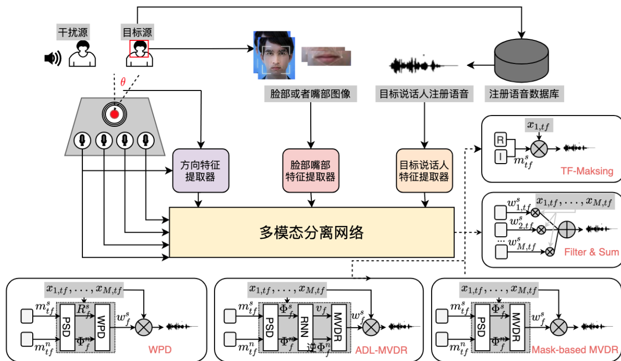
麦克风阵列分离的通用框架
