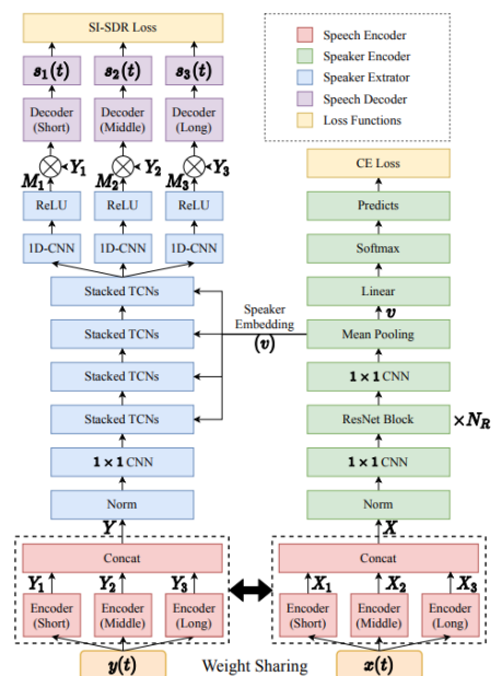
SpEx+框架
