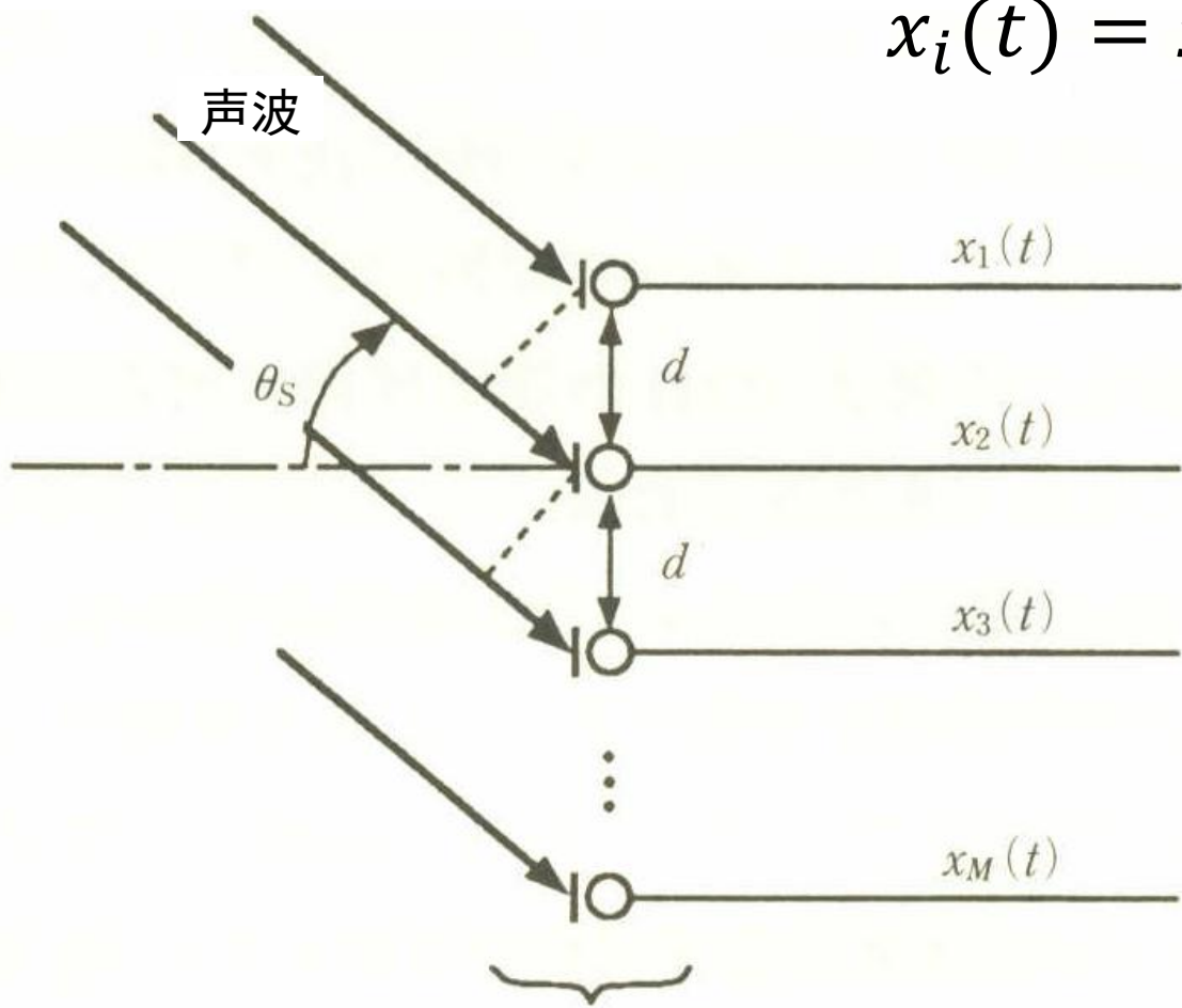
麦克风阵列
