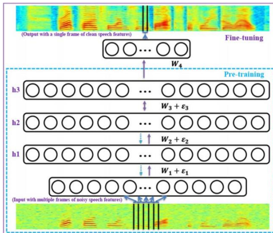
映射模型示意图
