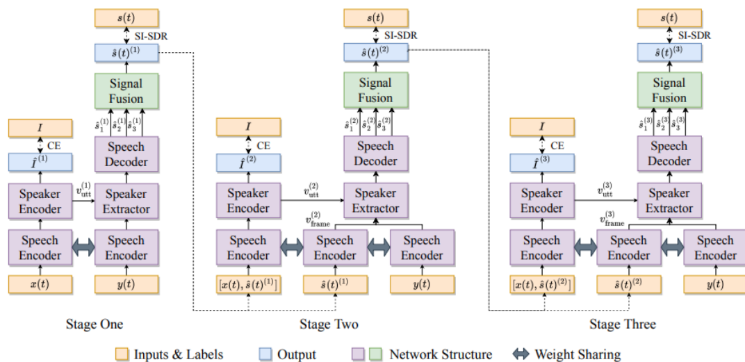
SpEx++框架
