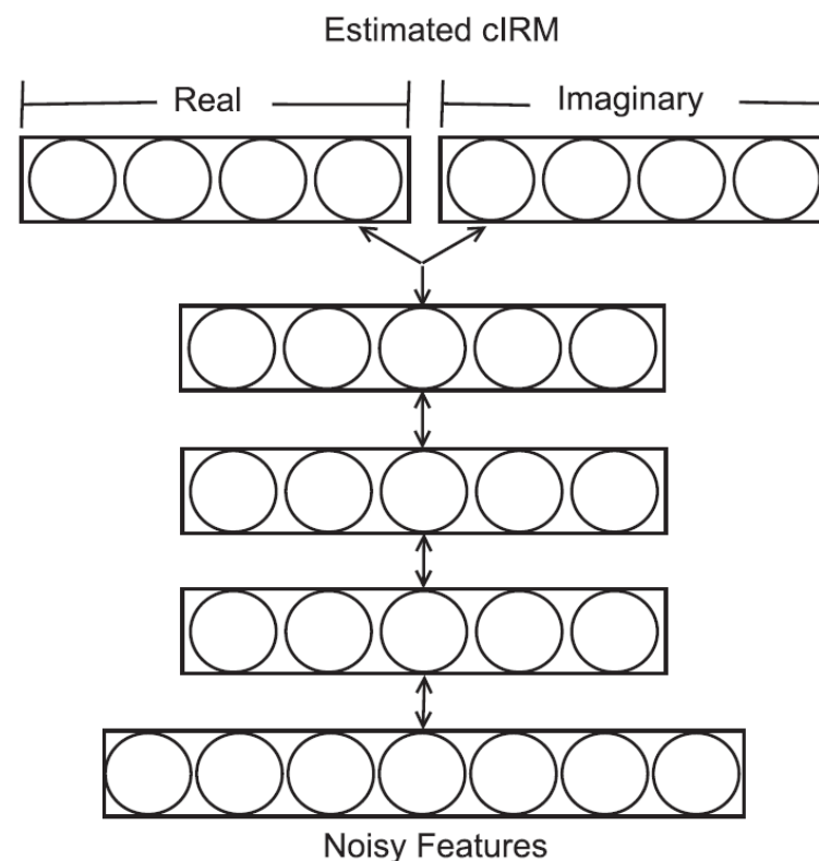
cIRM的DNN结构
