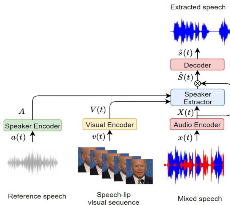
视听多模态分离的通用框架
