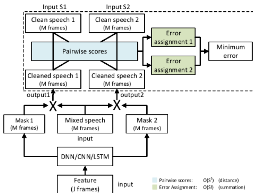
自下而上的PIT分离框架
